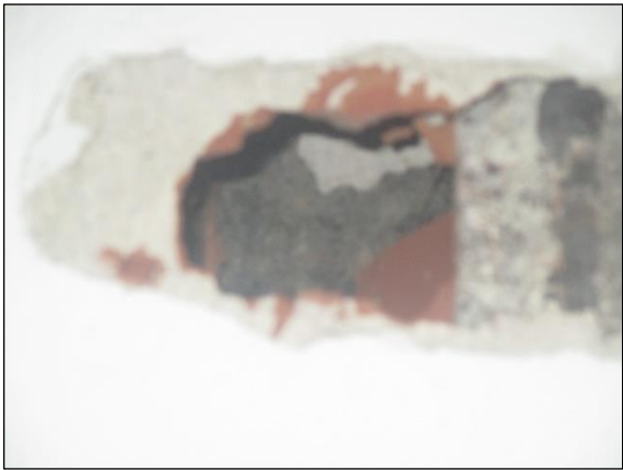
Foto n°2 - Particolare del profilo metallico utilizzato come elemento portante del solaio.
