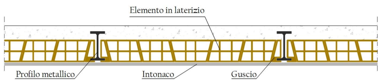
Disegno n°3 - Schematizzazione dell'andamento della sezione della Tipologia Solaio 1.
