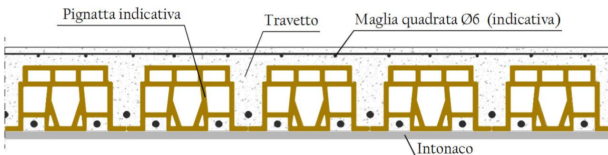
Disegno n°4 - Schematizzazione dell'andamento della sezione della Tipologia Solaio 2.
